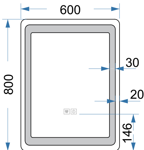
Pohled zřepředu Front view
