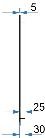
Boční pohled Side view
